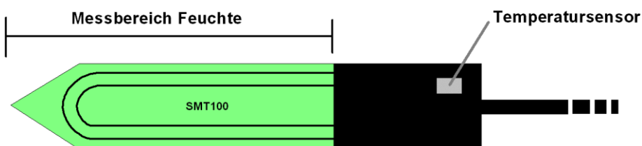
Bild 2: Skizze des Sensors SMT100 mit grüner kapazitiver Messfläche und Position des Temperatursensors
